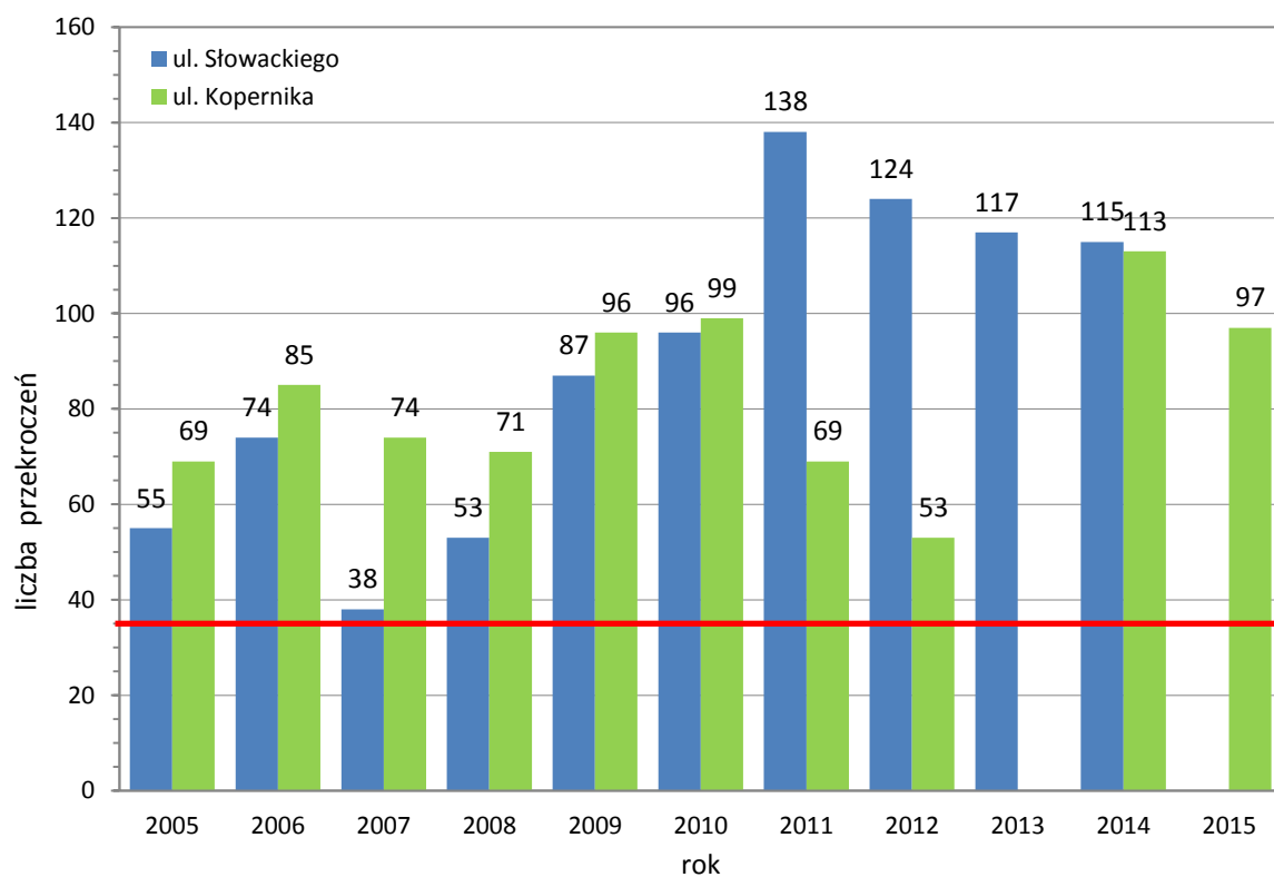
Rys. F. 6 Częstość przekraczania dopuszczalnego poziomu stężeń 24-godzinnych pyłu zawieszonego PM10 w latach 2005-2015 w powiecie żywieckim na podstawie pomiarów na stacjach monitoringu w Żywcu
