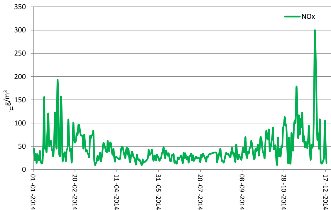
Rys. T. 21 24-godzinne stężenia NOx na stacji pomiarowej w Żywcu przy ul. Słowackiego
