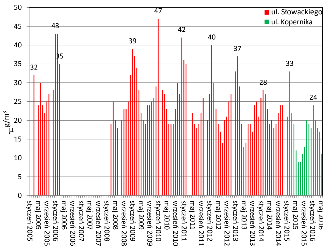
Rys. P. 18 Średnie miesięczne stężenia NO 2 w powiecie żywieckim na podstawie pomiarów na stacjach monitoringu powietrza w Żywcu w latach 2005-2016
